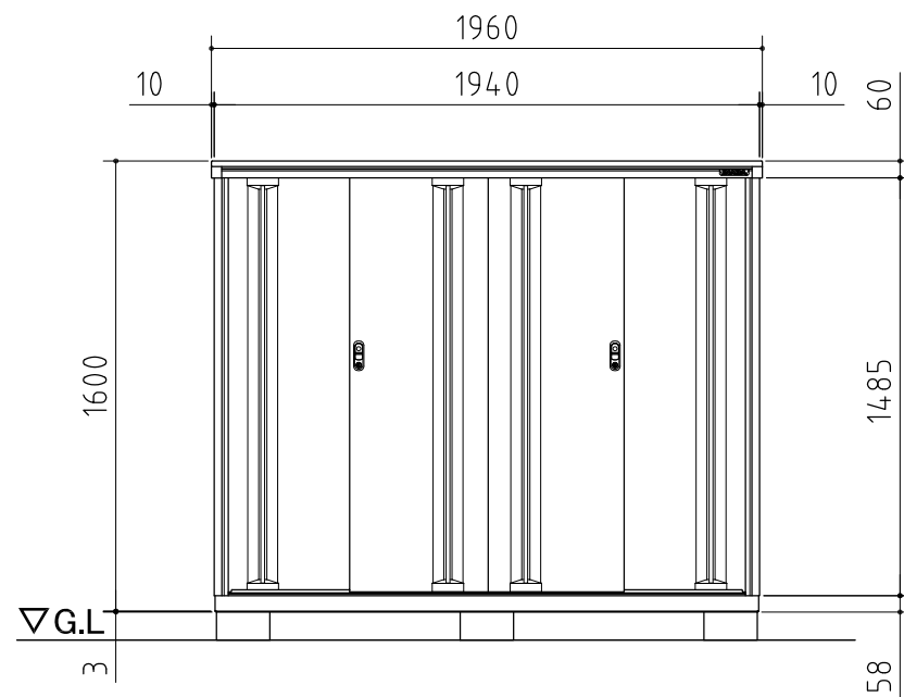
正面図
